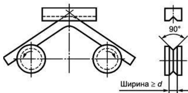
Рисунок Б.1 - Схема устройства для изгиба
