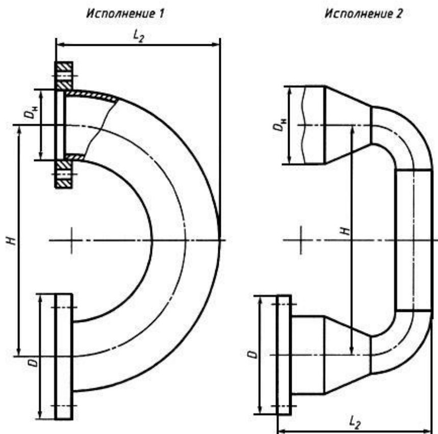
Рисунок 10 - Калач соединительный
