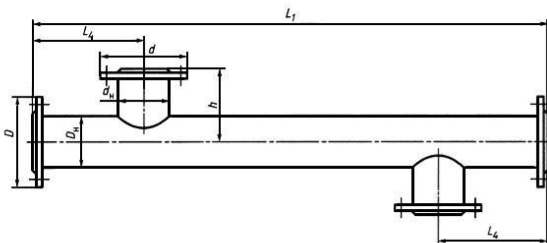
Рисунок 4 - Подогреватель из четырех блоков-секций типа ПВ2К с типовым расположением патрубков с компенсатором на корпусе
